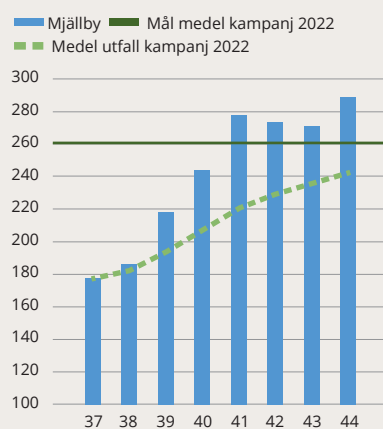
Mjällby medelproduktion (ton hst/dygn).
